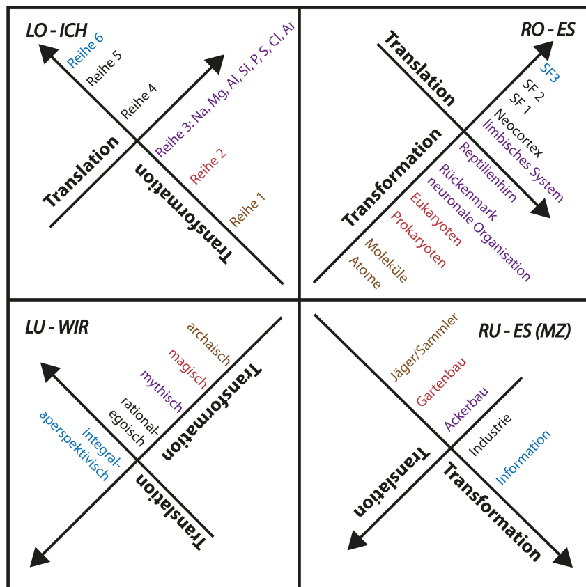
Abbildung 5: Transformation und Translation in den vier Quadranten
