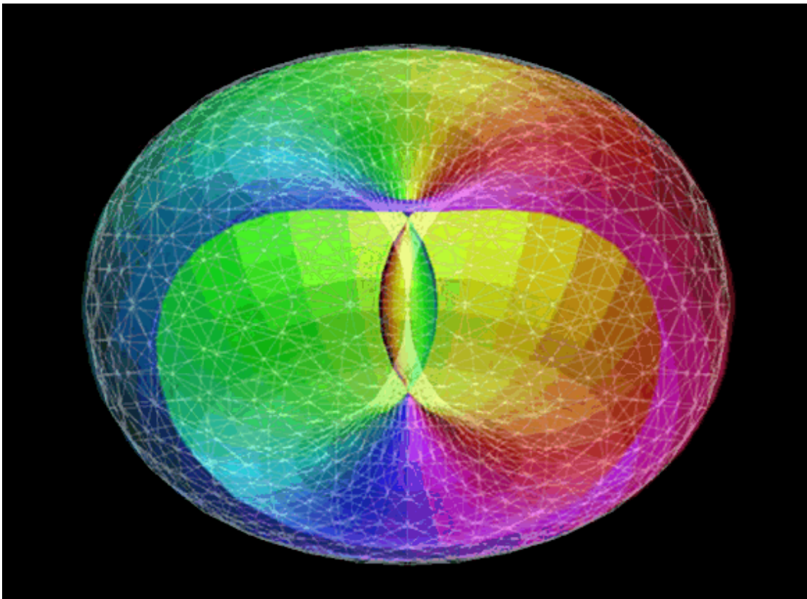
Abbildung 2: dreidimensionales Pulsieren in einem Torus.
